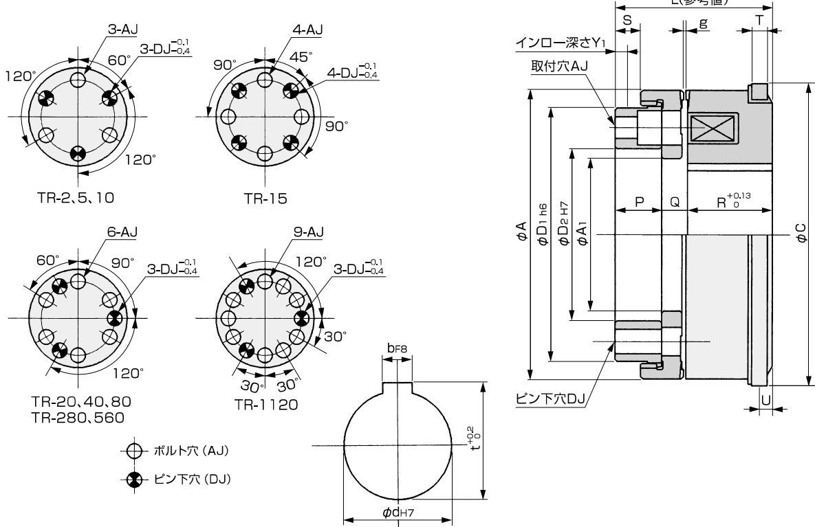
スプラインアダプタ取付穴位置
